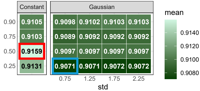
FDR
