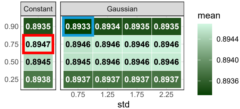
Precision
