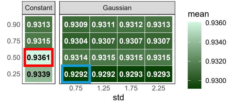
NPV
