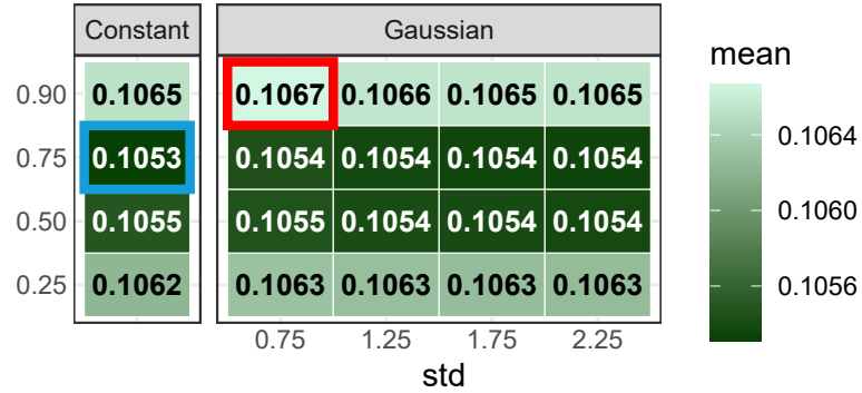
Precision
